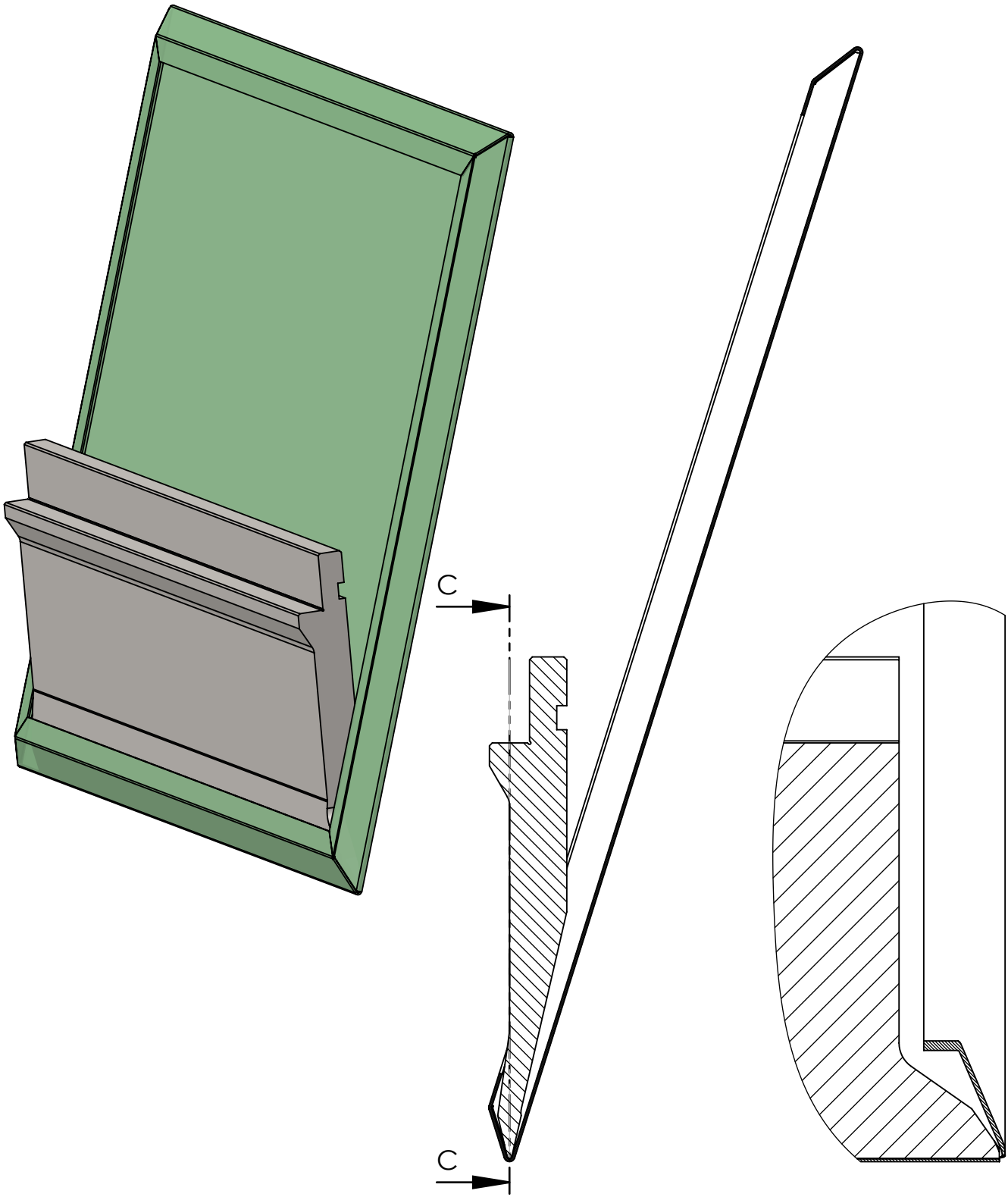
SEZIONE C-C
